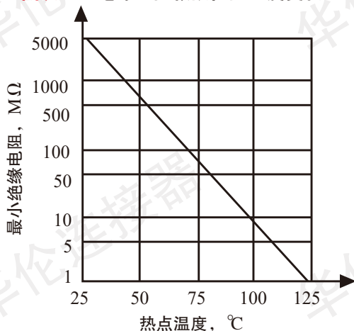
图A 绝缘电阻极限值随温度变化
