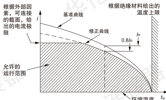
额定值下降曲线
