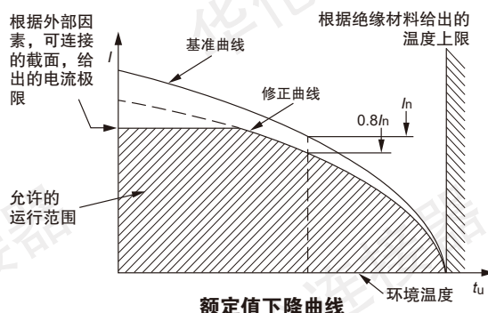
额定值下降曲线
