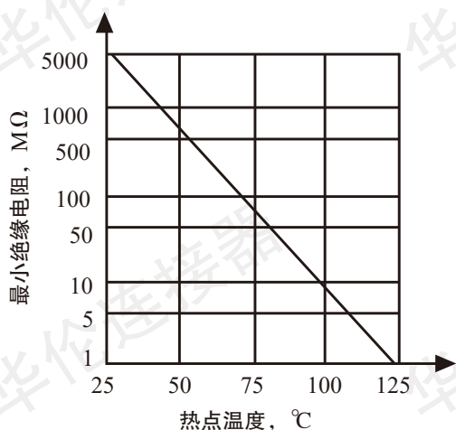
图表A 绝缘电阻极限值随温度变化
